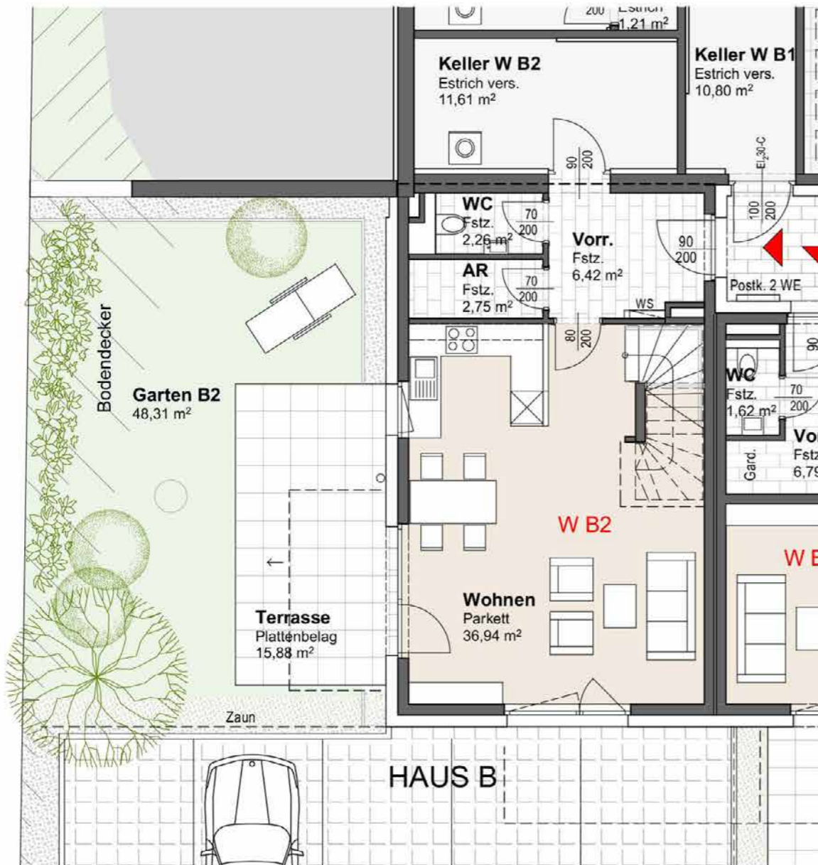
Ebene 0
