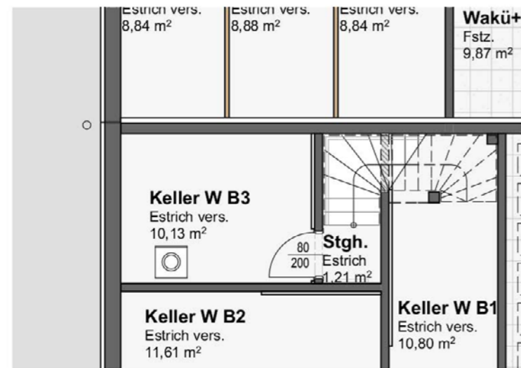
Ebene 0
