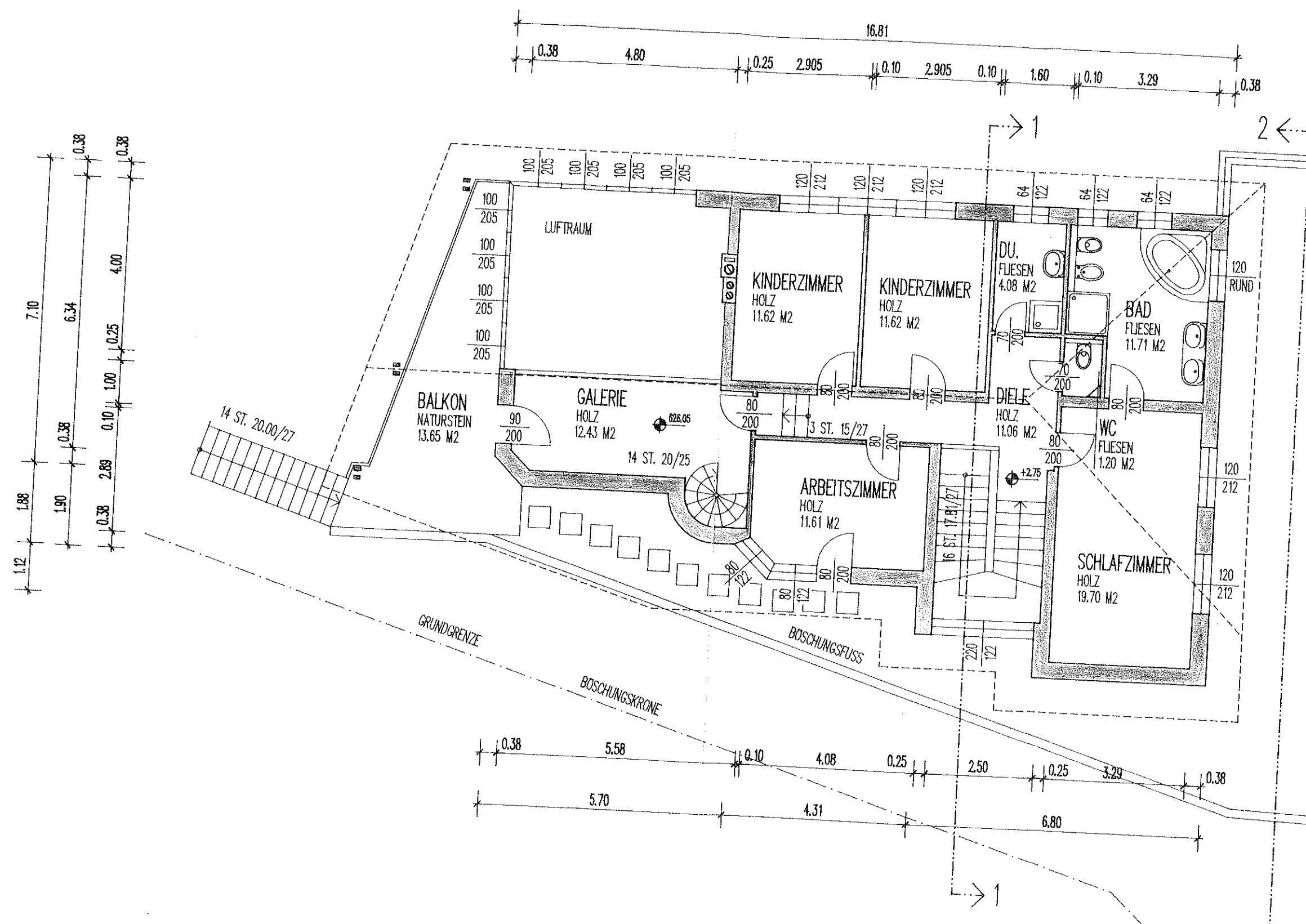
GRUNDRISS OBERGESCHOSS M 1:100
