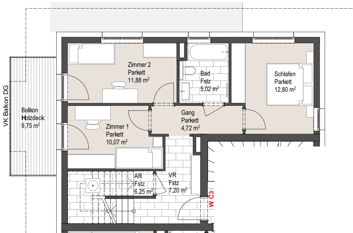
Wohnung C3 - Obergeschoss
